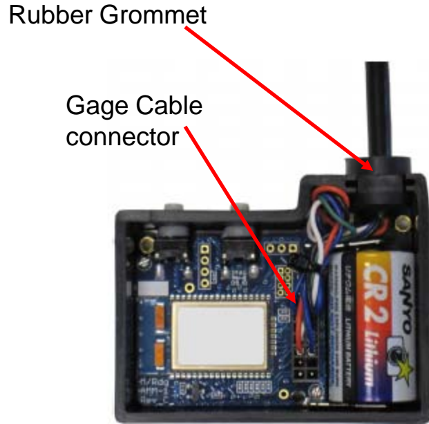
Mobile Module Gage Cable
